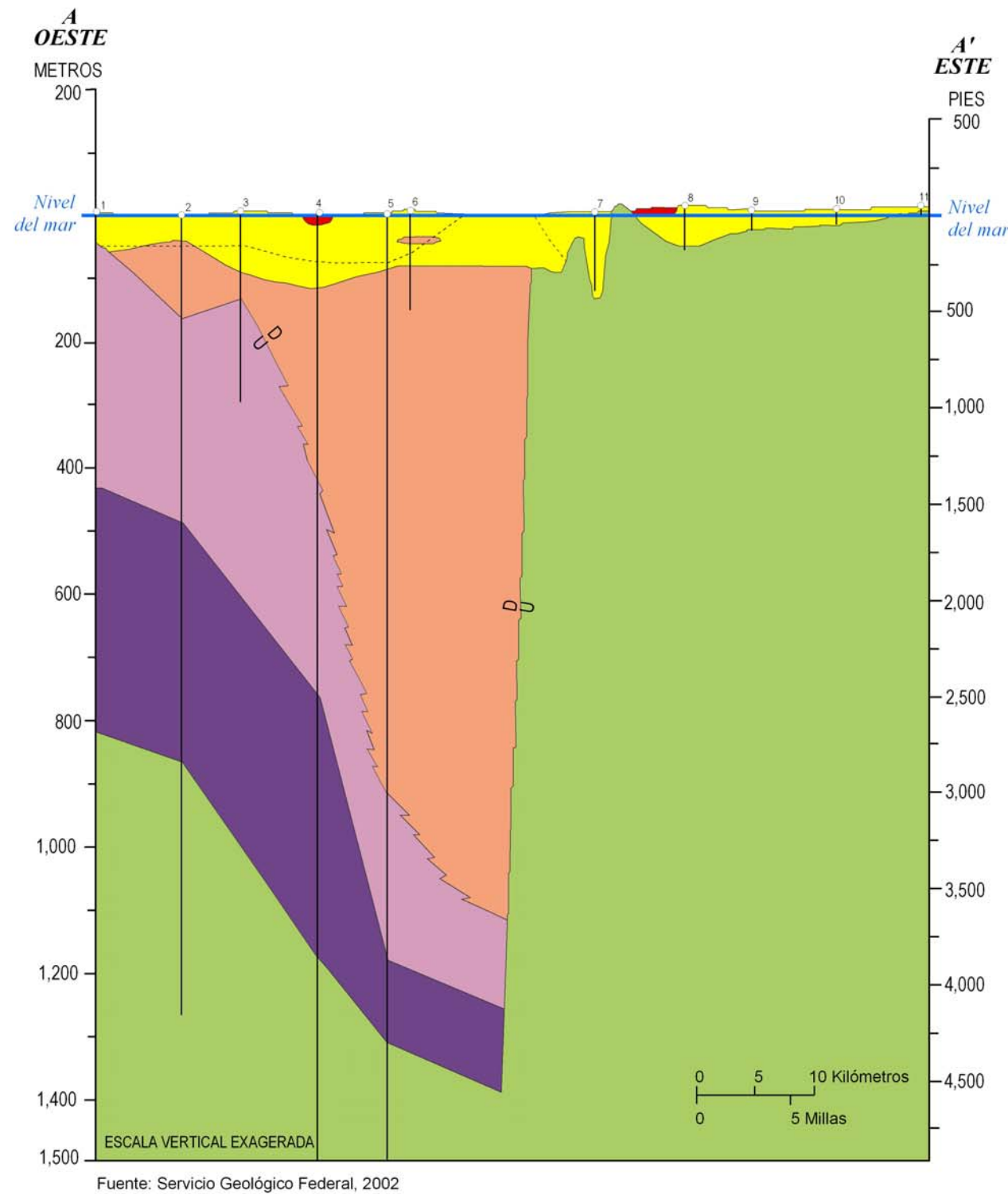
Figura 3-6. Sección geológica generalizada de la Región Sur de Puerto Rico (modificado de Renken, 2002, (Refiérase a la Figura 3-6 para localización)).
