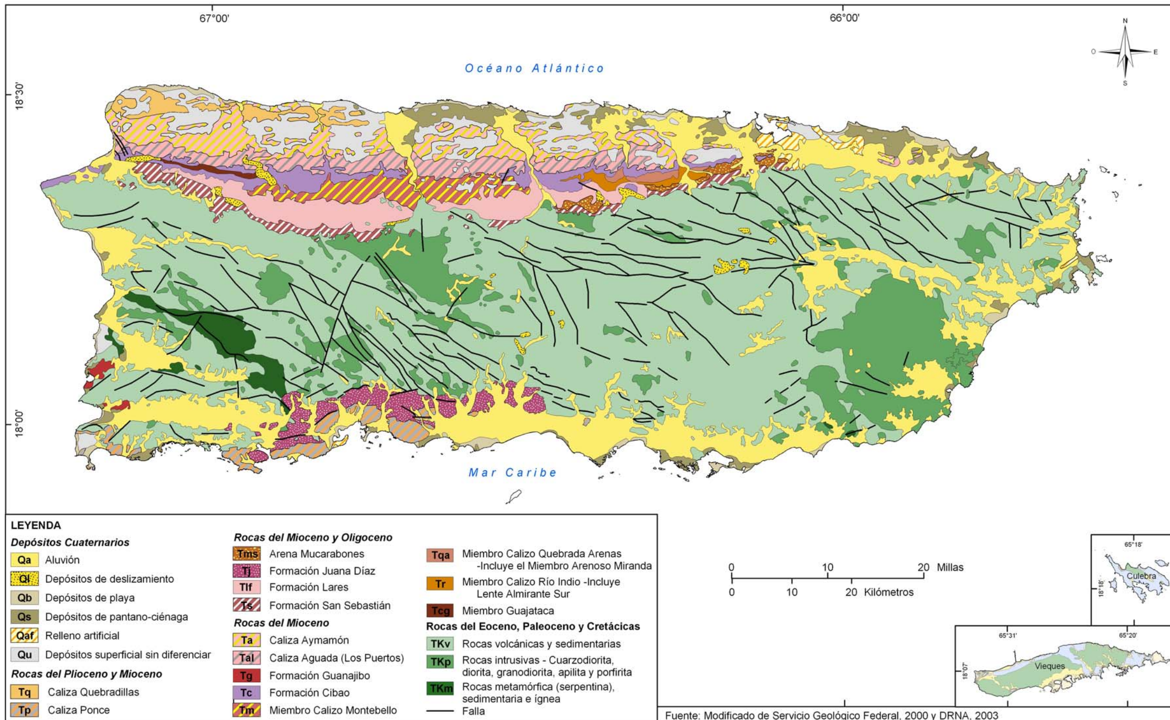
Figura 3-1. Mapa generalizado de la geología de Puerto Rico.
